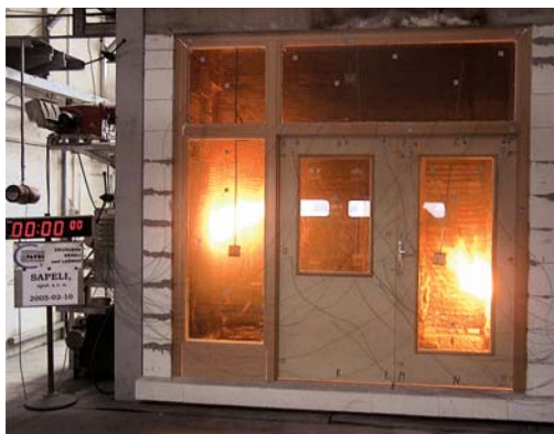
zkouška požární odolnosti – začátek
