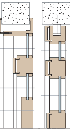
řez obložkovou zárubní řez rámovou zárubní
