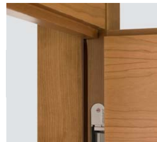
detail napojení dveří a nadsvětlíku
