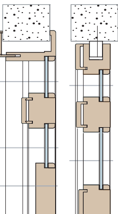
řez obložkovou zárubní
